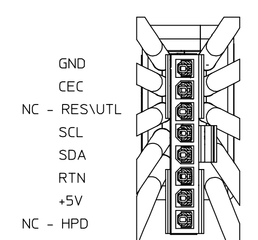
DETAIL B - SCALE 2:1 SCALE 2:1
