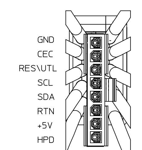
DETAIL B - SCALE 2:1 SCALE 2:1
